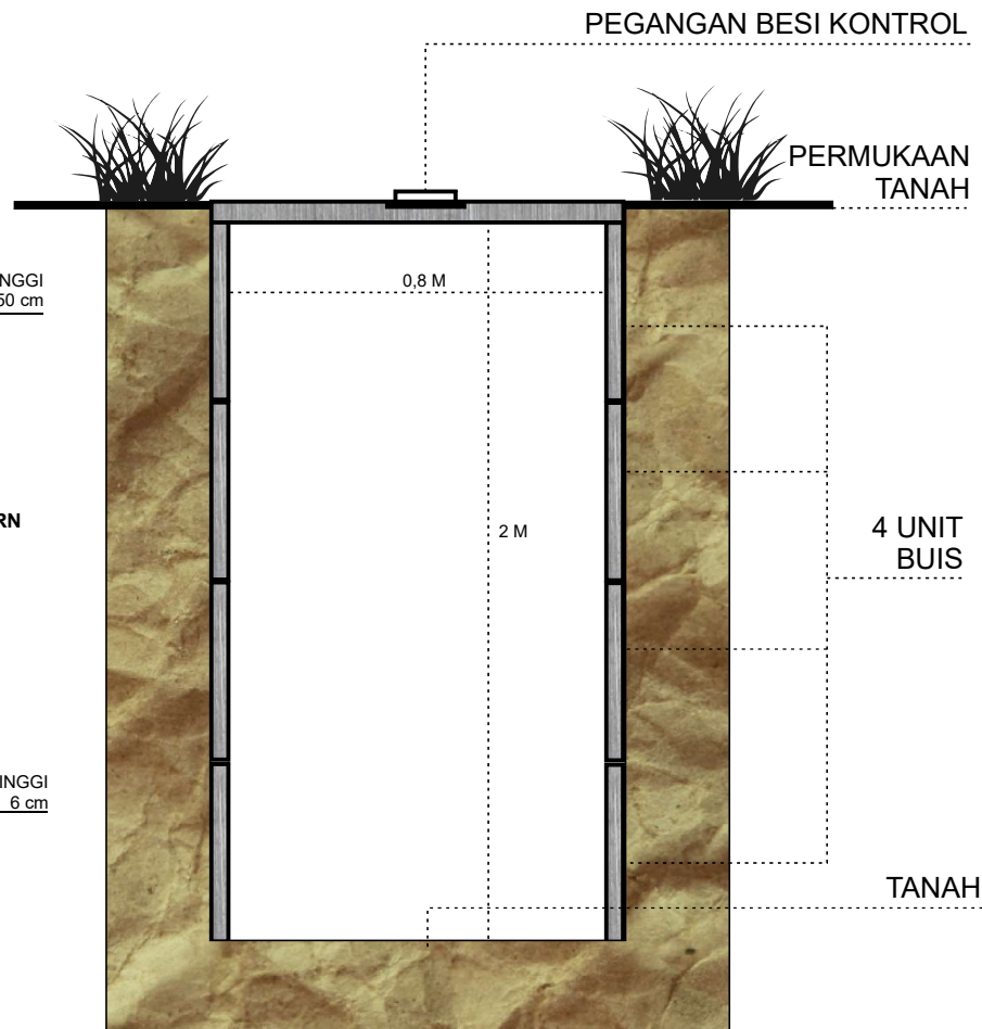
GAMBAR 5. PEMASANGAN BUIS / TEBA MODERN Skala 1 : nts
