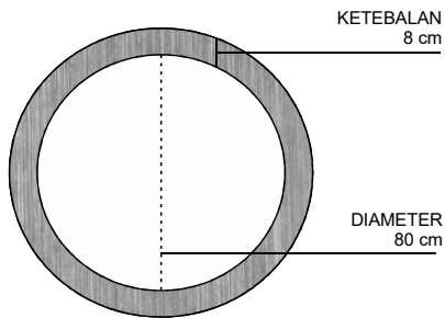
GAMBAR 1. TAMPAK ATAS BUIS TEBA MODERN Skala 1 : nts
